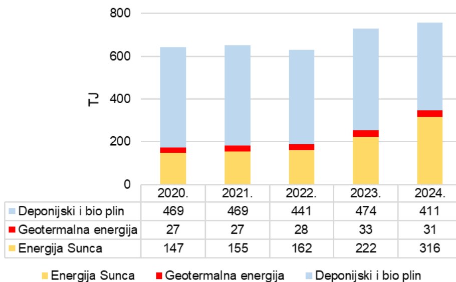
Slika 1.1. Proizvodnja primarne energije u Gradu Zagrebu za razdoblje od 2020. do 2024. godine
