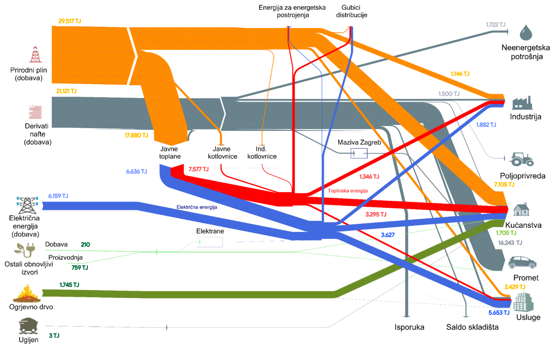
Slika 1.11. Shematski prikaz toka energetske bilance Grada Zagreba za 2024. godinu
